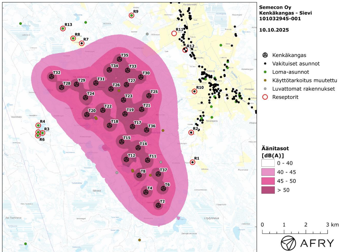
Kuva 3-2: Keskiäänitasot L_{Aeq} Kenkäkankaan tuulivoimapuiston hankealueella.
