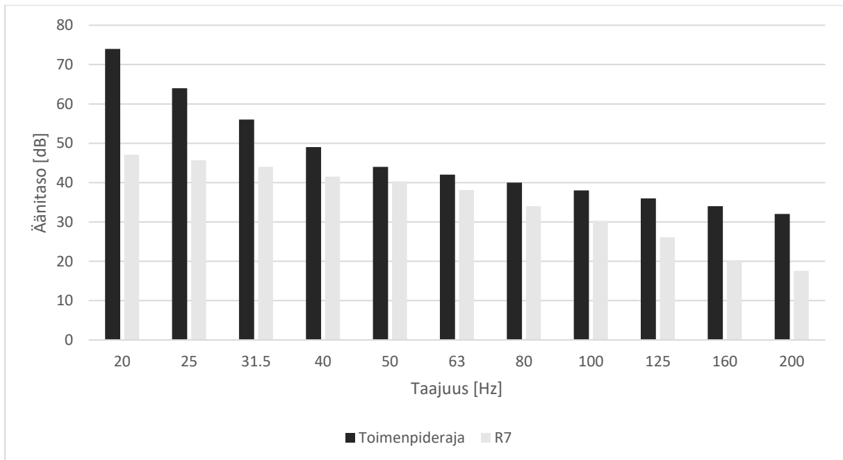
Kuva 3-3: Matalataajuisen sisämelun tasot reseptorin R7 kohdalla.
